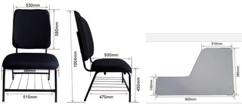
Dimensões para Assento, Encosto e Prancheta.
